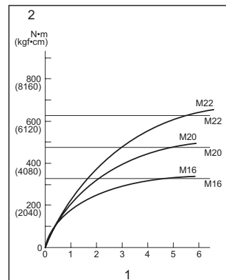
1. Timp de strângere (secunde) 2. Cuplu de strângere
