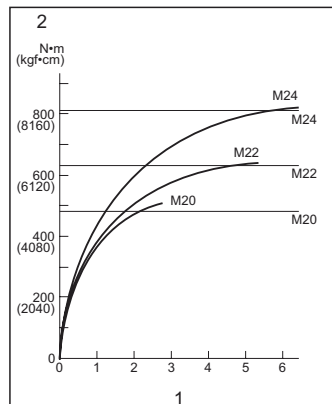
1. Час затягування (с) 2. Момент затягування
