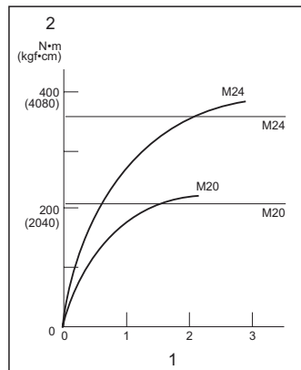
1. Czas dokręcenia (s) 2. Moment dokręcenia
