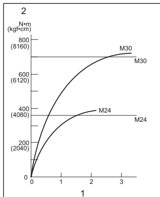
1. Meghúzási idő (másodperc) 2. Meghúzási nyomatóka
