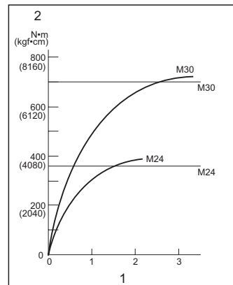
1. Czas dokręcania (s) 2. Moment dokręcenia
